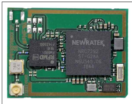
일본 실렉스가 지난 4월 초 출시한 장거리 와이파이 모듈 (TELEC 최초 인증) (제품명 : SX-NEWAH)
